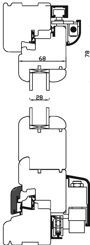
Sezione B-B'
