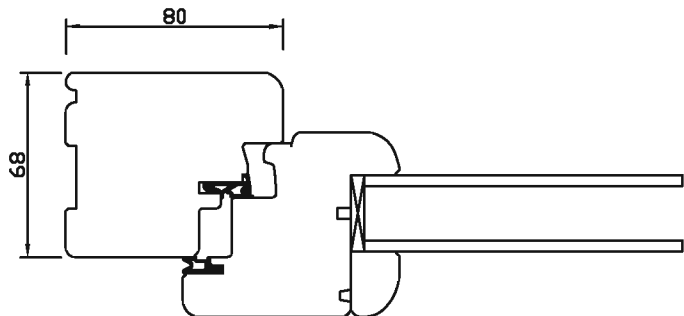
Sezione A-A'
