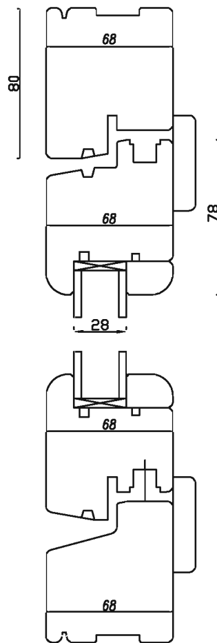
Sezione B-B'
