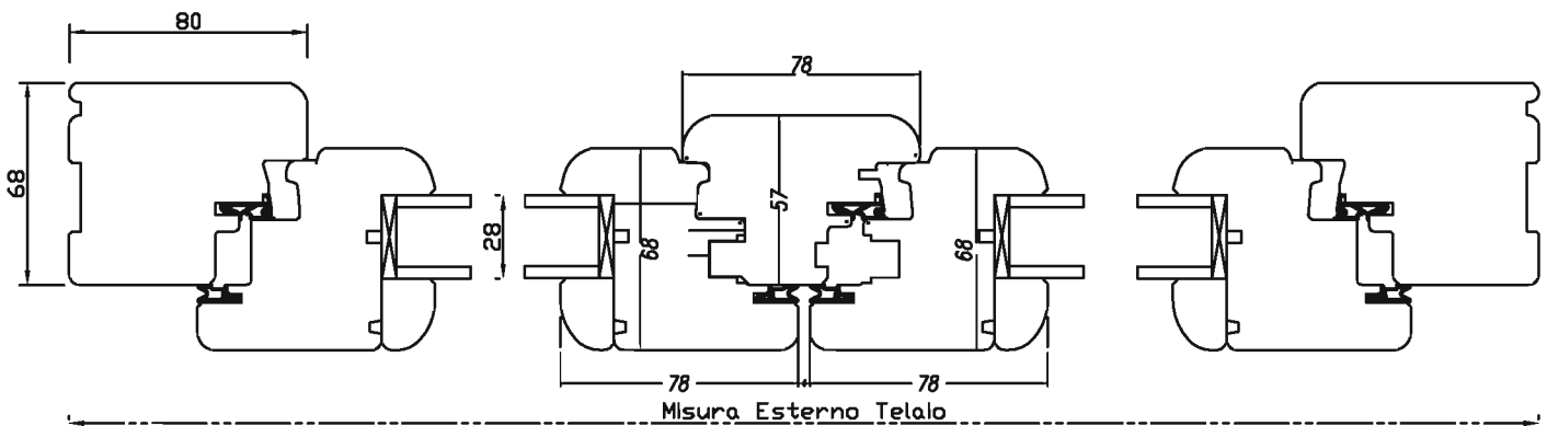
Sezione A-A'
