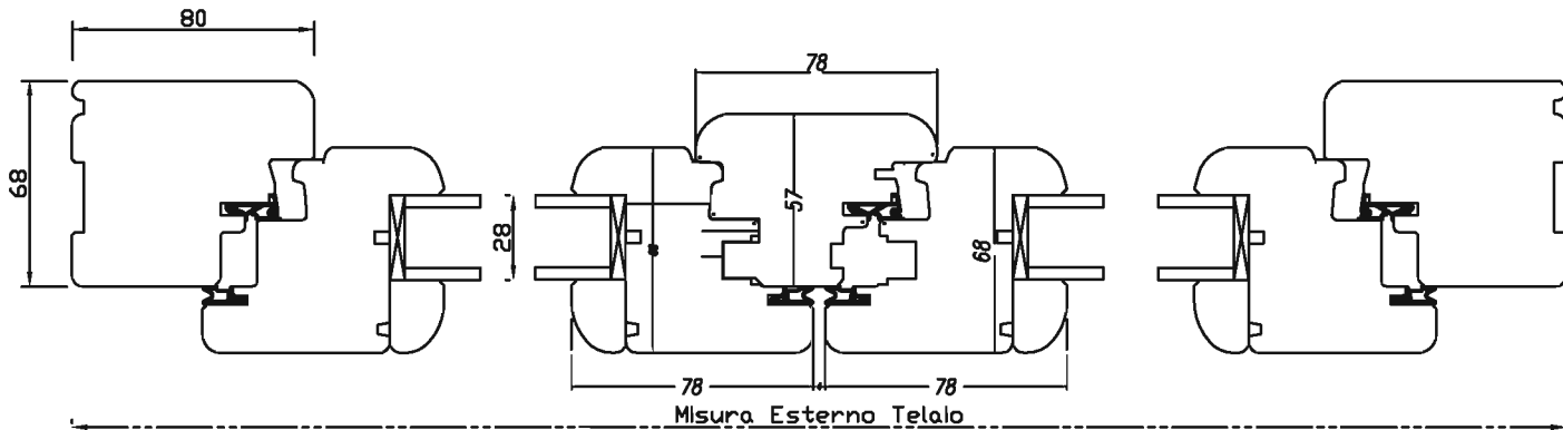
Sezione A-A'
