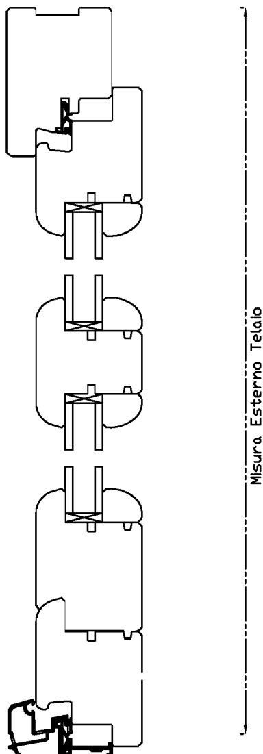
Sezione B-B'
