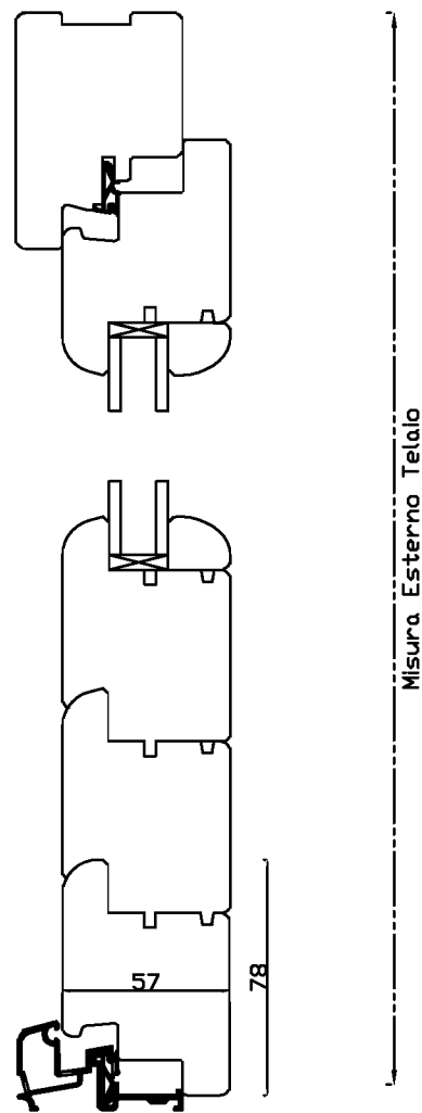
Sezione B-B'
