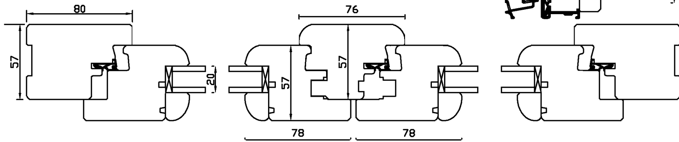
Sezione A-A'
