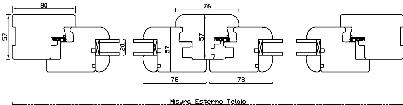
Sezione A-A'
