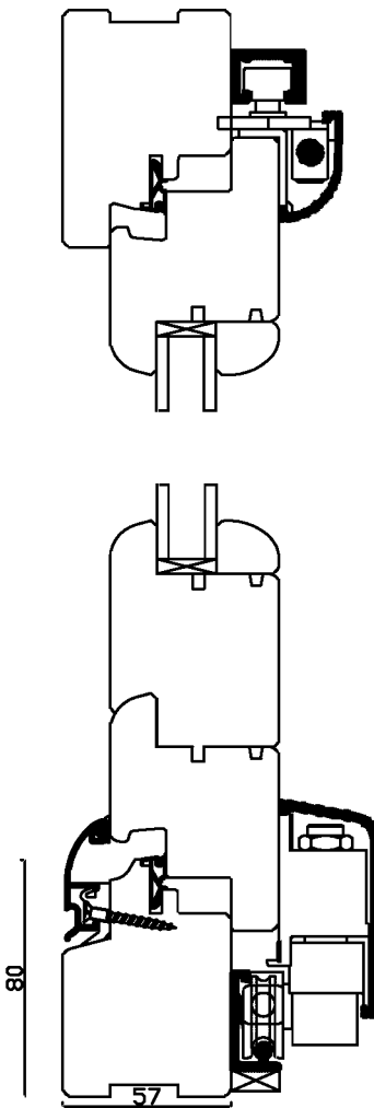
Sezione B-B'
